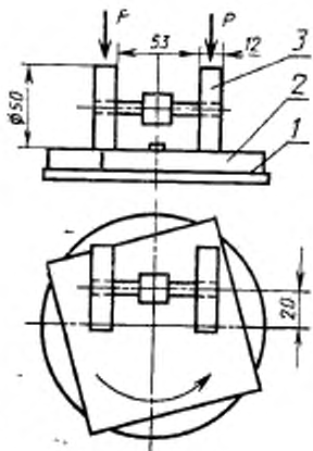
Схема прибора для определения стойкости покрытий к истиранию
