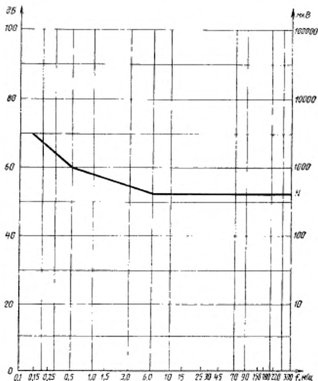
Характеристика допустимых величин радиопомех
