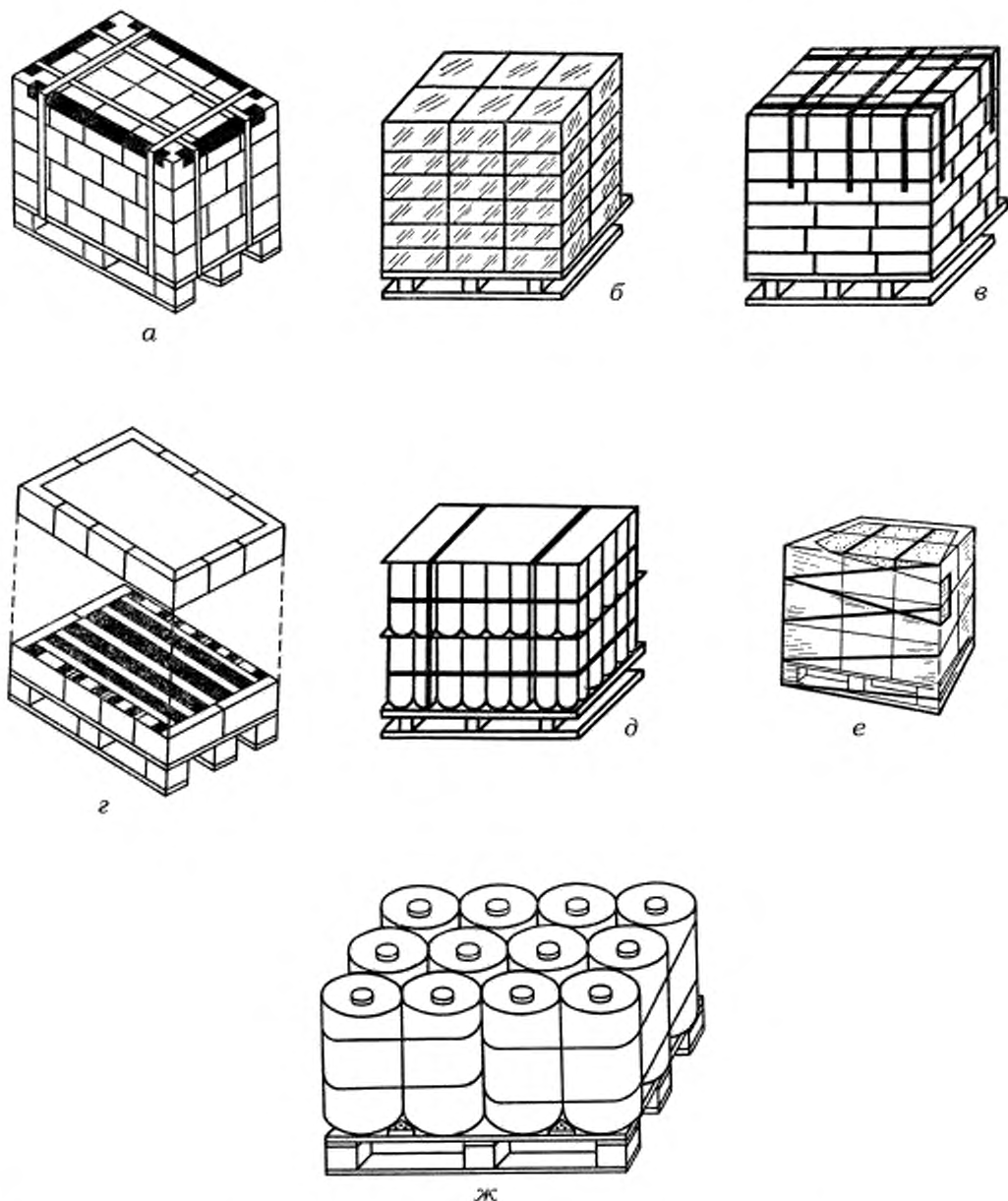
a — скрепление при помощи клея, ленты и уголков; б — скрепление пакетирующей пленкой; в — скрепление клейкой лентой; г — скрепление при помощи клея и крафт-бумаги; д — скрепление проволокой с применением картонных прокладок; е — скрепление при помощи растягивающейся пленки; ж — скрепление барабанов на поддоне
