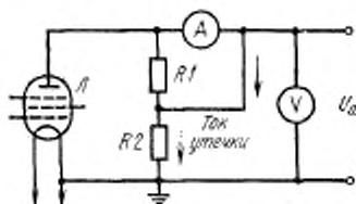
Л—лампа, А—амперметр, V—вольтметр, R1—сопротивление току утечки через охлаждающую воду.
