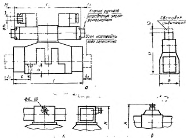
Размеры, мм
