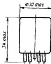
Расположение штырьков РШ-24 по ГОСТ 7842—71
