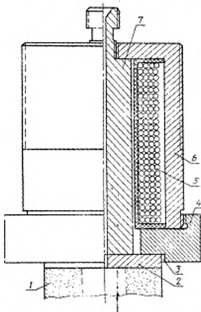
Схема магнитного захвата
