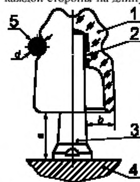
1 — изолятор; 2 — уплотнитель; 3 — штырь; 4 — траверса; 5 — проводник; а — расстояние от нижнего края юбки до траверсы; б — расстояние от края юбки до штыря; д — диаметр проводника
