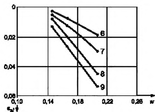
в) График зависимости относительной просадочности от влажности
