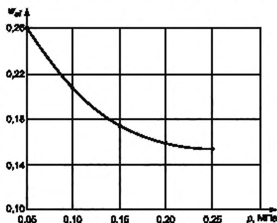
б) График зависимости начальной просадочной влажности w_{sj} от давления p
