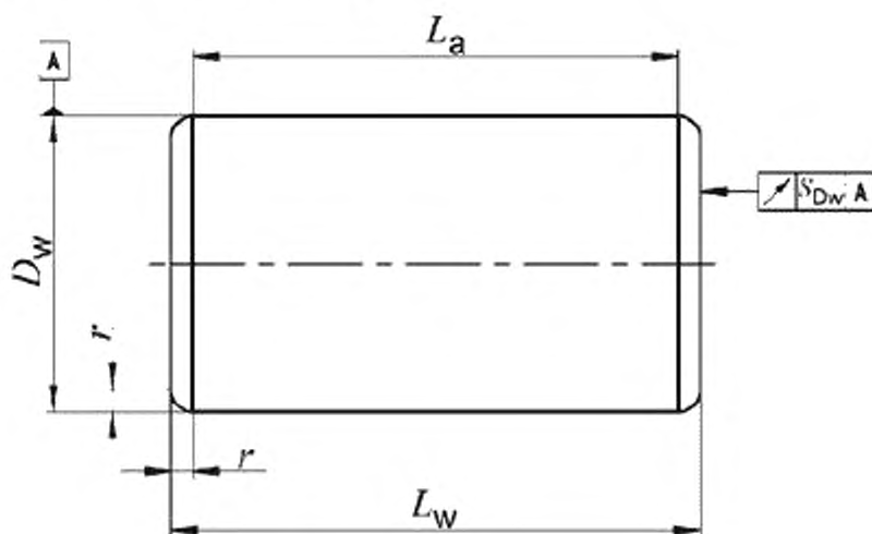
Рисунок 1 – Цилиндрический ролик
