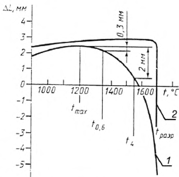
1 – для алюмосиликатных огнеупоров; 2 – для периклазовых огнеупоров.
