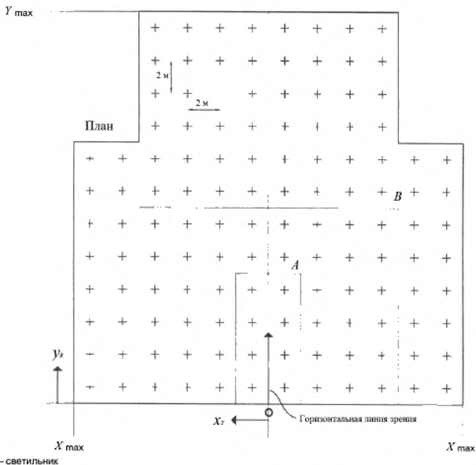
Рисунок 3 — Стандартное расположение светильников в плане по [3] (площадь A соответствует размерам 2H x 4H, площадь B соответствует размерам 8H x 6H)
