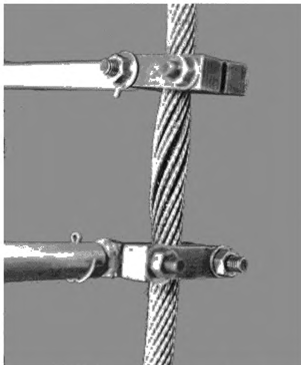
Рисунок Б.1 — Прямолинейный участок каната
