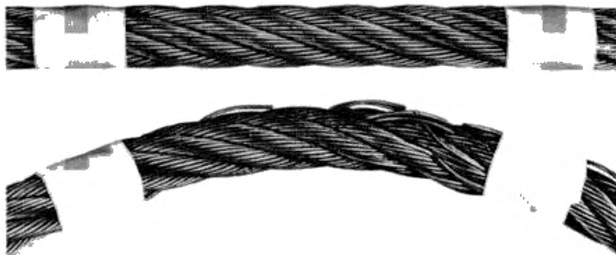
Рисунок 7 — Обрывы проволок в углублениях между прядями каната
