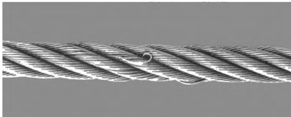
Рисунок А.1 — Выдавливание проволоки из пряди
