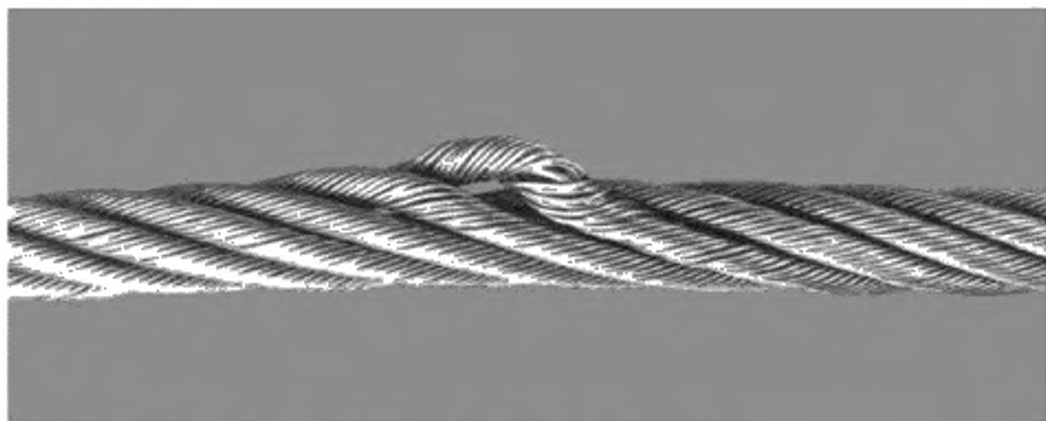
Рисунок А.4 — Выдавливание пряди
