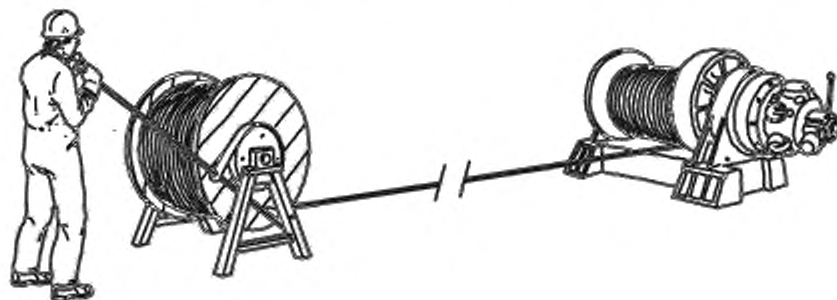
Рисунок 3 — Многослойная навивка каната с бобины на барабан лебедки
