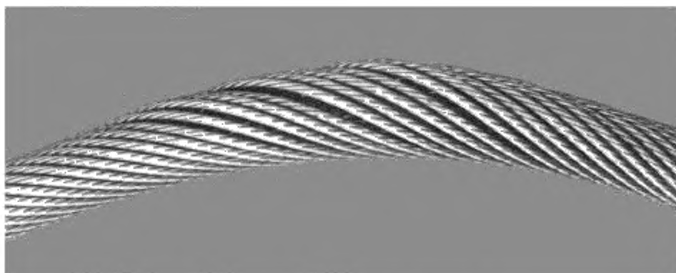
Рисунок А.9 — Корзинообразная деформация
