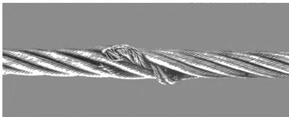
Рисунок А.2 — Выдавливание сердечника
