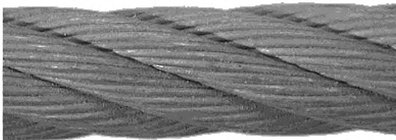
Рисунок Ж.1 — Начало окисления каната (следы коррозии). Коррозию можно удалить протиркой. Степень повреждения — 0 %
