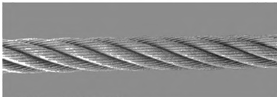
Рисунок А.11— Наружная коррозия
