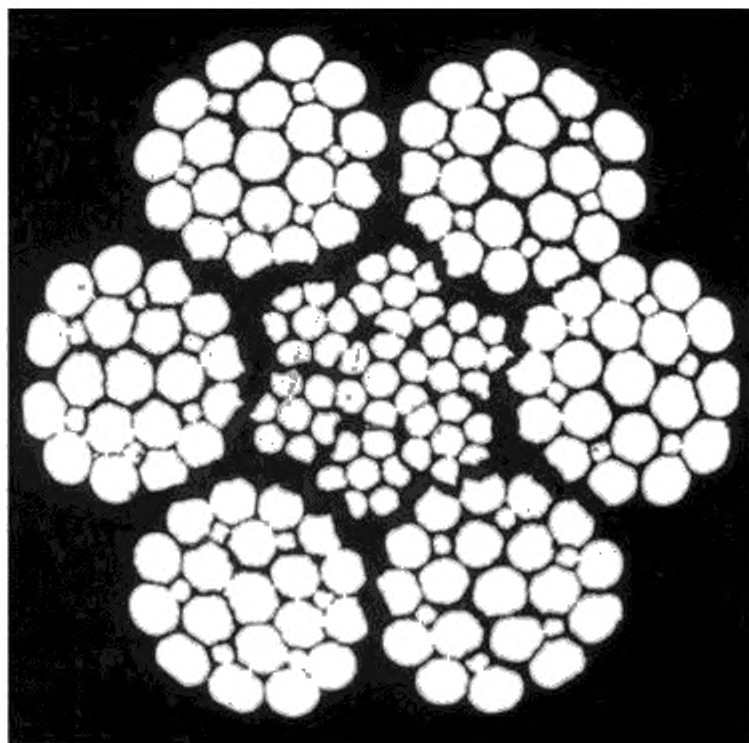
Рисунок А.19 — Внутренняя коррозия
