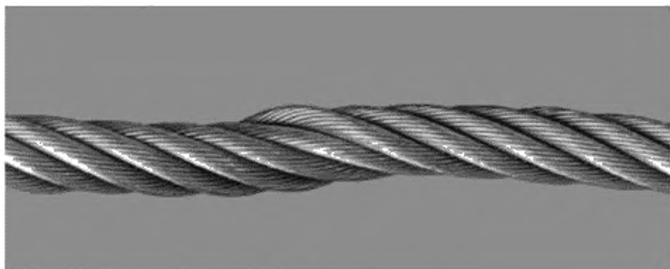
Рисунок А.6 — Перекручивание каната
