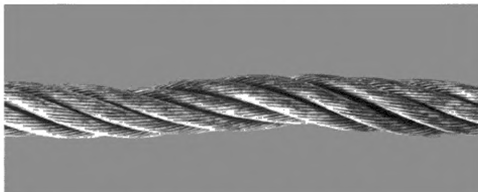
Рисунок А.3 — Местное уменьшение диаметра каната
