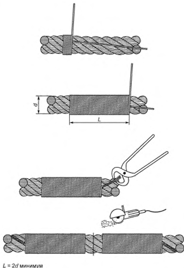
Рисунок 4 — Обвязка каната перед отрезанием
