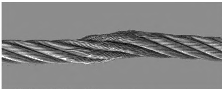
Рисунок А.7 — Раскручивание каната
