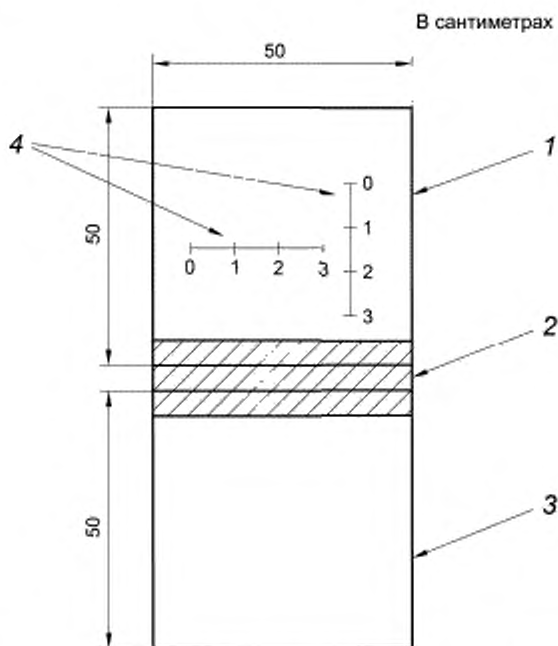
1 — откалиброванный слайд из стекла; 2 — лента из клейкой ленты; 3 — покровное стекло, 4 — шкалы для подсчета ячеек
