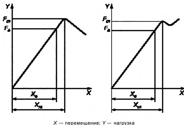
Рисунок 2 — Пример кривой «нагрузка — перемещение» для режима В
