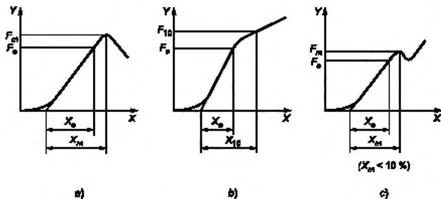
Рисунок 1 — Пример кривой «нагрузка — перемещение» для режима А
