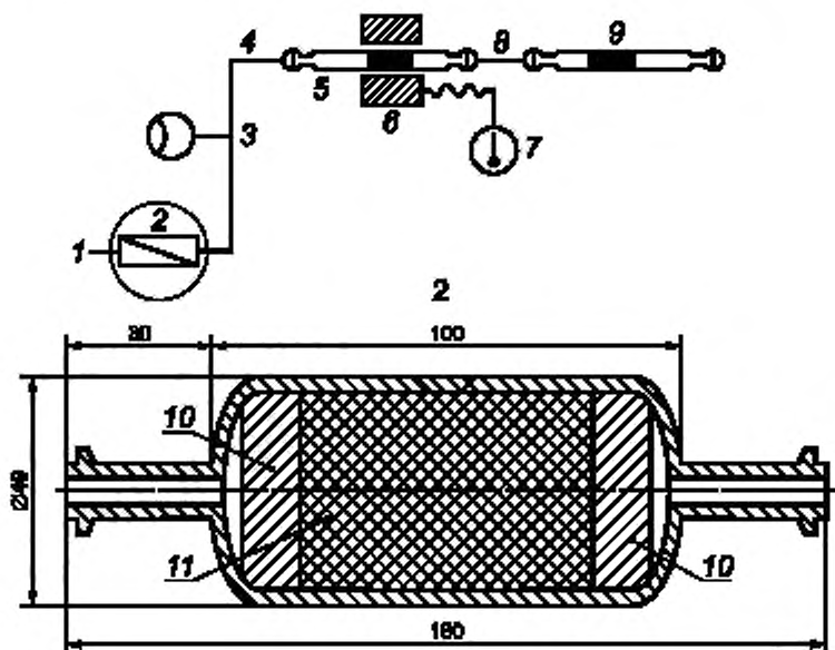
1 — воздушный насос; 2 — ловушка для ртути; 3 — ротаметр; 4 — трубки из ПВА; 5 — пробоборная трубка; 6 — лед для трубок; 7 — термометр; 8 — соединительная стеклянная трубка; 9 — аналитическая трубка; 10 — стекловолокно; 11 — адсорбент (например, активированный уголь, обработанный серой)
