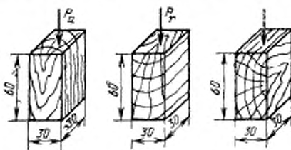
a - (P_a) — нагрузка, сжимающая образец вдоль волокон, b - (P_b) — нагрузка, сжимающая образец поперек волокон в радиальном направлении, z - (P_z) — нагрузка, сжимающая образец поперек волокон в тангентальном направлении
