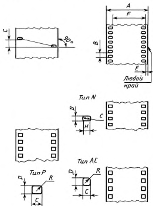
Типы перфораций
