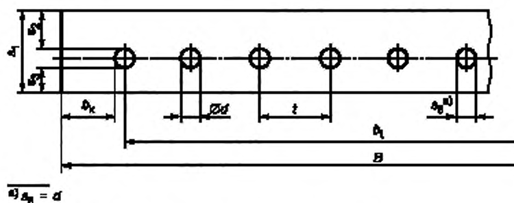
Рисунок 1 — Поперечное сечение стандартной ленты
