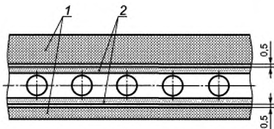
1 — обкладки; 2 — поперечное армирование
